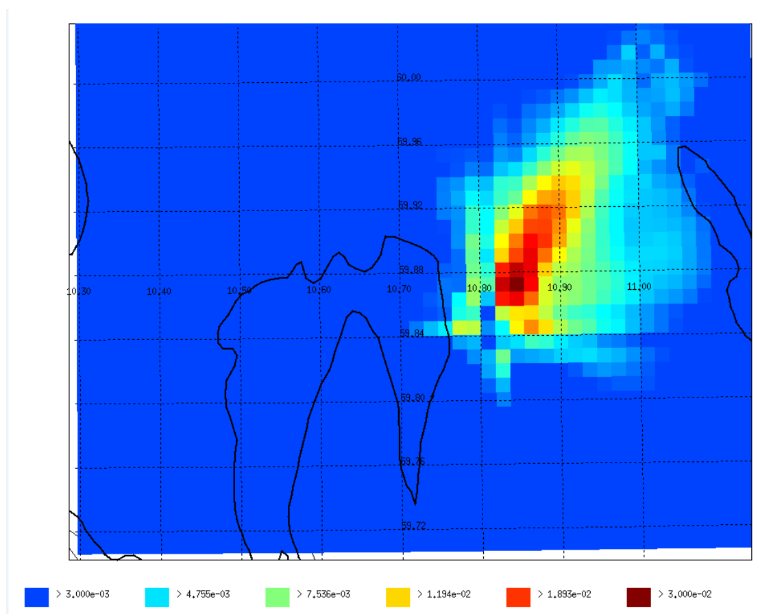
Figur 3: Årlig gjennomsnitt av SO 2 bakkekonsentrasjon (µg SO 2 /m 3 ) beregnet med WRF-EMEP-modellen med oppløsning 1 km for et utslipp på 1 g/s.
